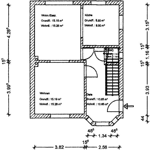
Erdgeschoss
