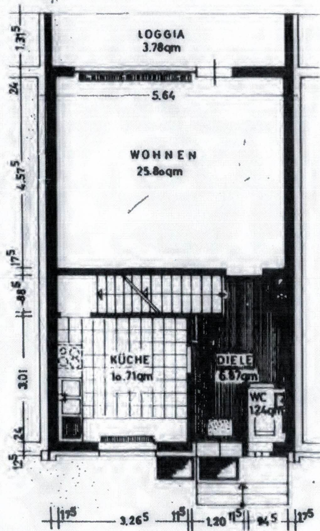
ERDGEOSCHOSS
