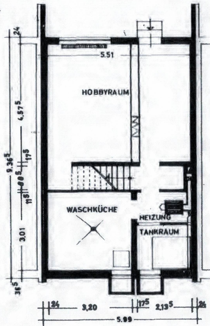
KELLERGEOSCHOSS
