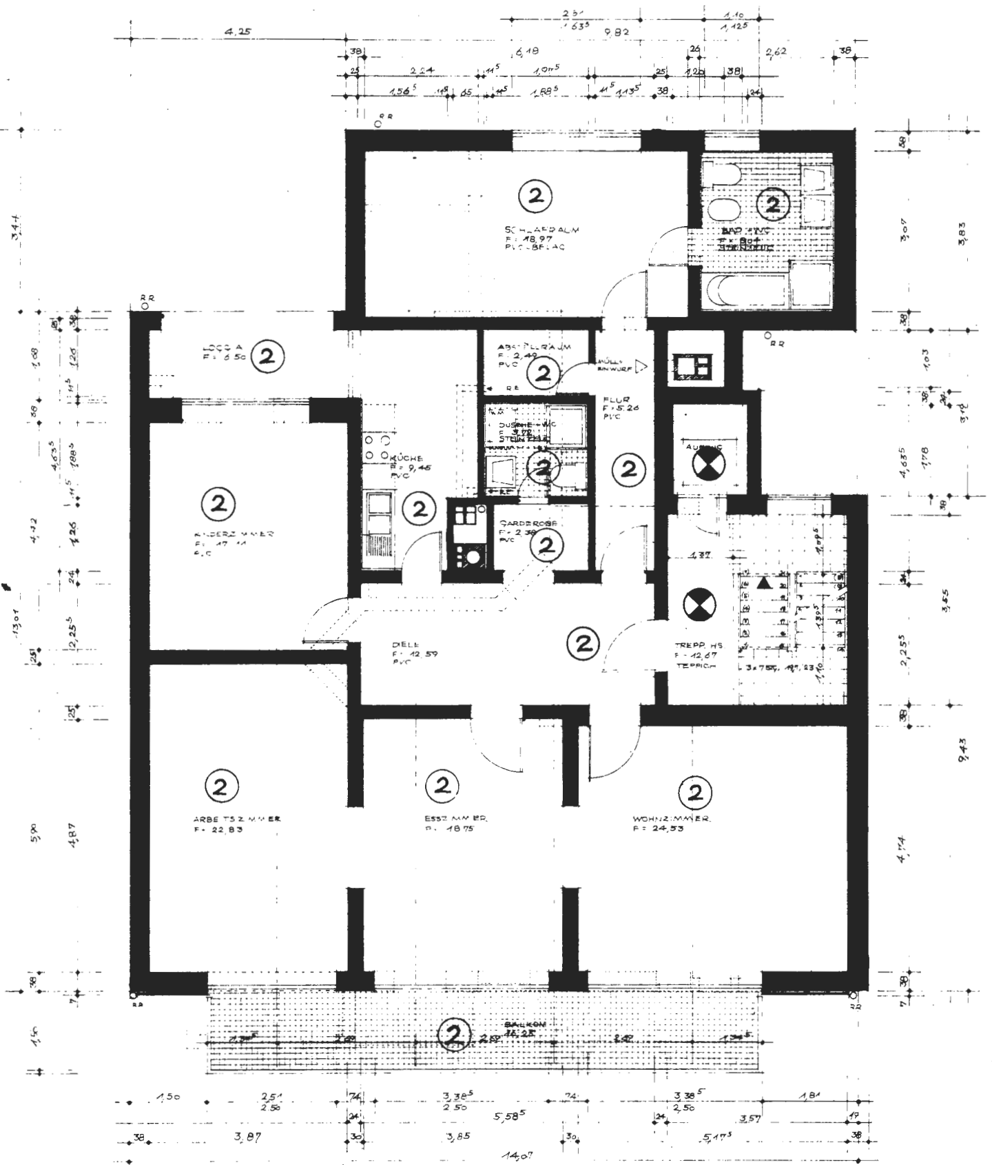
1. OBERGESCHOSS
